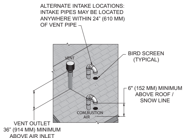
Figure 5-1B Terminaisons verticales d'apport d'air et d'évacuation en acier inoxydable
