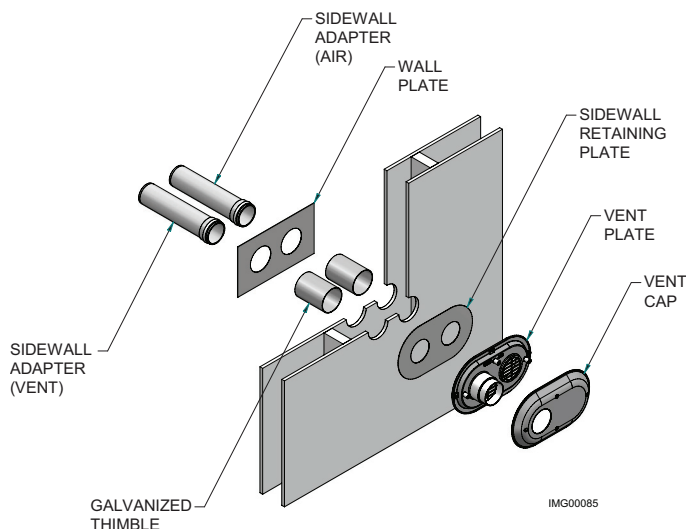
Figure 4-5B Terminaison murale en polypropylène
