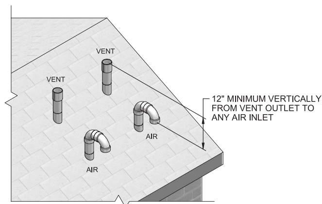
Figure 5-3 Terminaisons verticales optionnelles, plusieurs chauffe-eau
