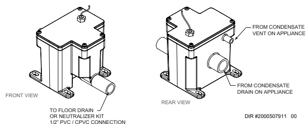
Figure 13 Collecteur de condensation
