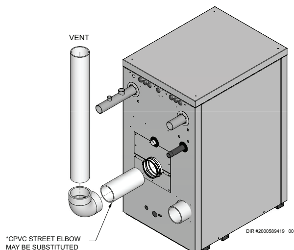
Figure 3-7 Tuyauterie d'évacuation en PVC/CPVC à proximité du chauffe-eau - Modèles 400 - 1000
