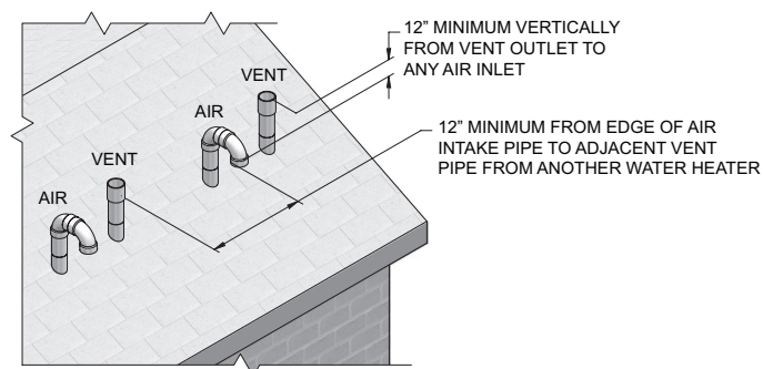
Figure 5-3 Terminaisons verticales optionnelles, plusieurs chauffe-eau
