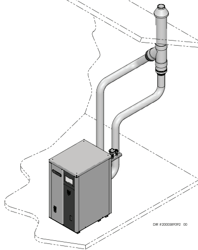
Figure 3-4 Terminaison concentrique verticale en PVC/CPVC
